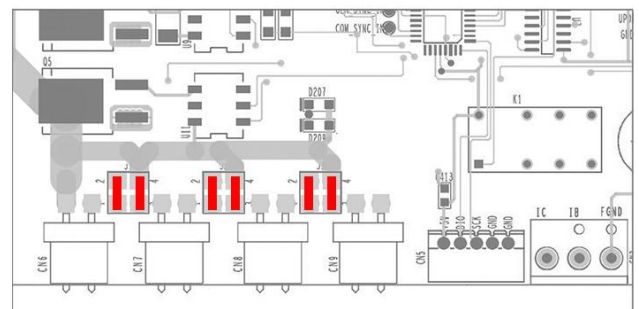
220/127 V 연결 방법
