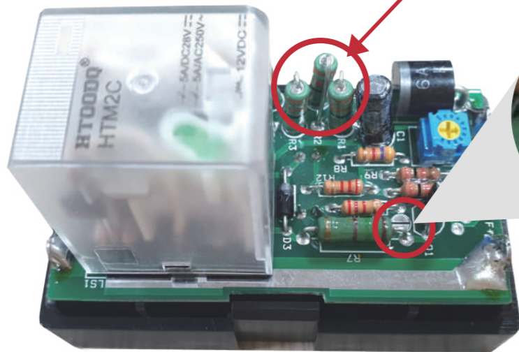
FFD-BF1 내부사진
